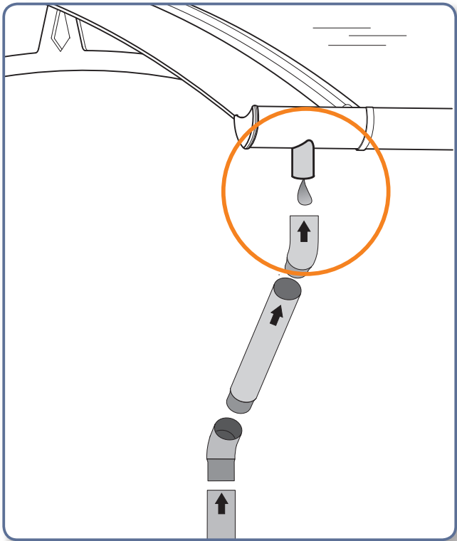
Predisposizione a tubazioni di scolo - Predisposition for draining pipes
