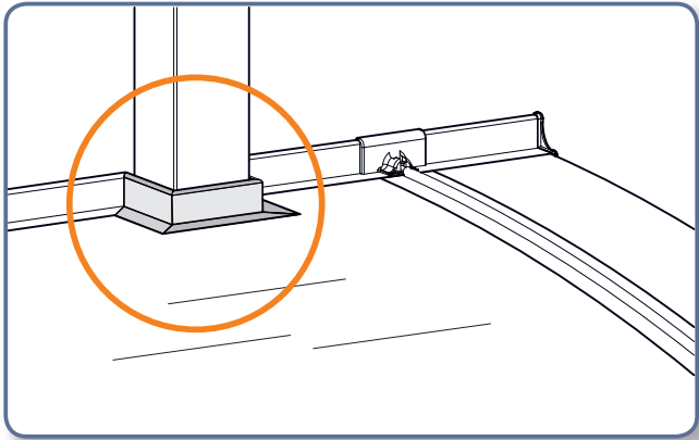
Passaggio tubi discendenti - Pipes crossing
