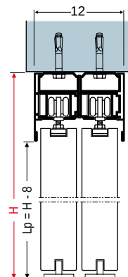
2As (due ante simmetriche) - 3As (tre ante simmetriche) - 4As (quattro ante simmetriche)
