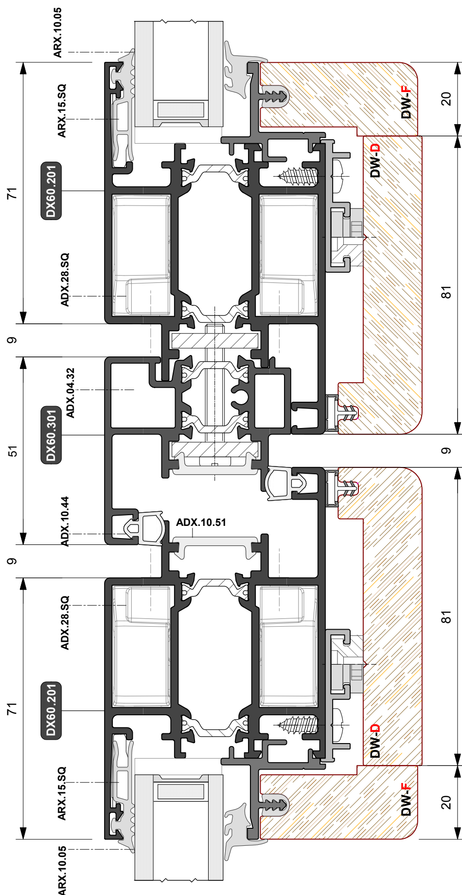
PORTA A DUE ANTE CON SOPRALUCE
