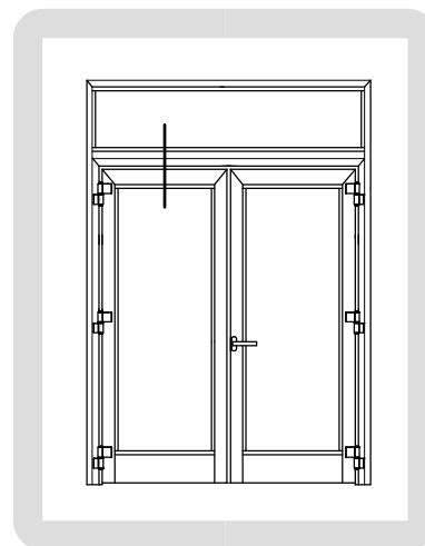
PORTA A DUE ANTE CON SOPRALUCE
